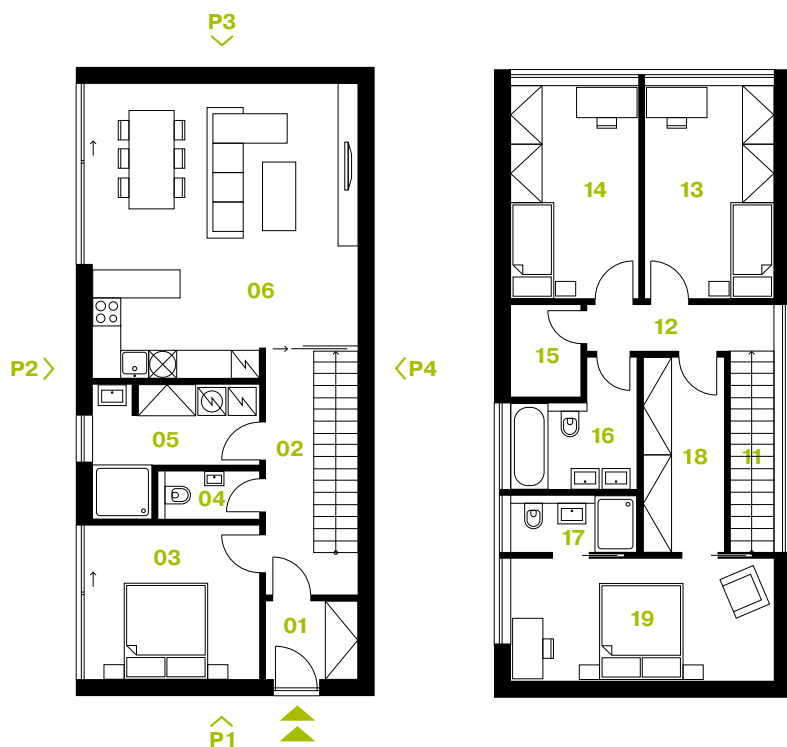
PŮDORYS PŘÍZEMÍ
