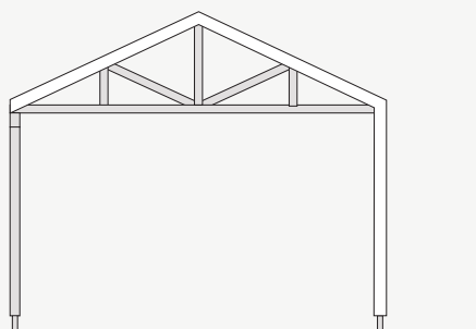
POHLED P4
